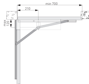
Corredero - DAB805PLA
