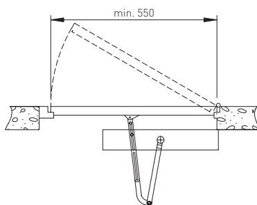
Articulado - SBA
