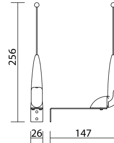
Dimensions R91/AN1/P1
